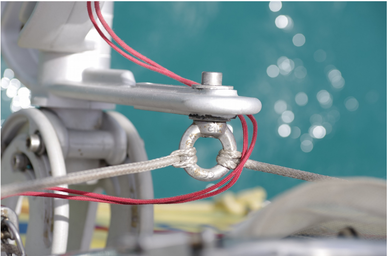
Fixation du bout qui relie le régulateur à la barre franche.
